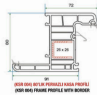
(KSR 004) 80'LIK PERVAZLI KASA PROFİLİ (KSR 004) FRAME PROFILE WITH BORDER
