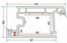
K 6005 KAPI KANAT PROFİLİ K 6005 DOOR SASH PROFILE
