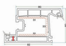
K 6022 BALKON KAPI KANAT PROFİLİ K 6022 BALCONY DOOR SASH PROFILE
