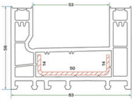
KSS 6101 SÜRME KASA PROFİLİ KSS 6101 SLIDING FRAME PROFILE
