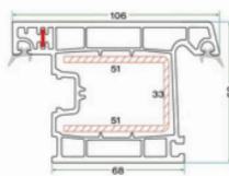
K 6016 DIŞA AÇILIR KAPI KANAT PROFİLİ K 6016 OUTWARD OPENING DOOR SASH PROFILE
