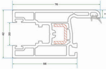
KES 002 SÜRME KANAT PROFİLİ KES 002 SLIDING SASH PROFILE
