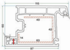
K 6005 KAPI KANAT PROFİLİ K 6005 DOOR SASH PROFILE
