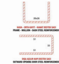
DIŞA AÇILIR KAPI DESTEK SAÇI OUTWARD OPENING DOOR STEEL REINFORCEMENT
