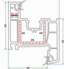
KYS 6003 KANAT PROFİLİ KYS 6003 SASH PROFILE
