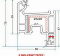
K 6004 KANAT PROFİLİ K 6004 SASH PROFILE
