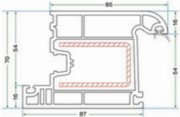
KRS 004 70'LIK KAPI PROFİLİ KRS 004 70 DOOR SASH PROFILE
