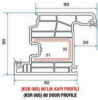
(KSR 005) 80'LIK KAPI PROFİLİ (KSR 005) 80 DOOR PROFILE
