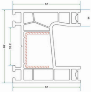
KES 001 SÜRME KASA PROFİLİ KES 001 SLIDING FRAME PROFILE
