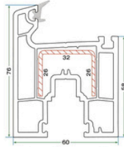
KSS 6102 SÜRME KANAT PROFİLİ KSS 6102 SLIDING SASH PROFILE
