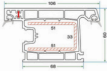
K 6016 DIŞA AÇILIR KAPI KANAT PROFİLİ K 6016 OUTWARD OPENING DOOR SASH PROFILE
